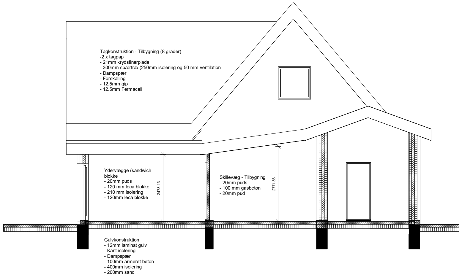
Section 4 1 : 50
