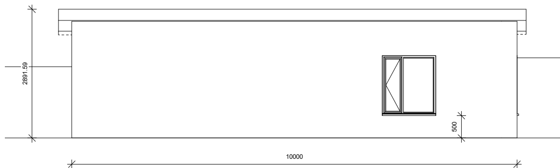
Garage Øst 1 : 50
