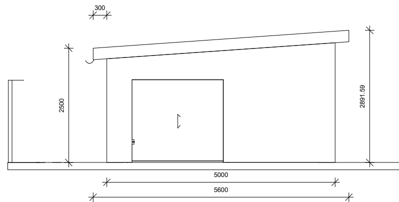
Garage Nord 1 : 50
