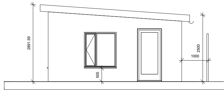
Garage Nord 1 : 50
